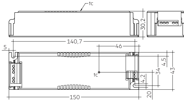
Ohne Zugentlastung
